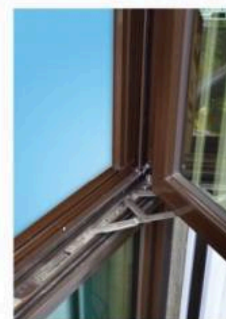
❷三點定位桿，可分三段式開啟所留開口。
